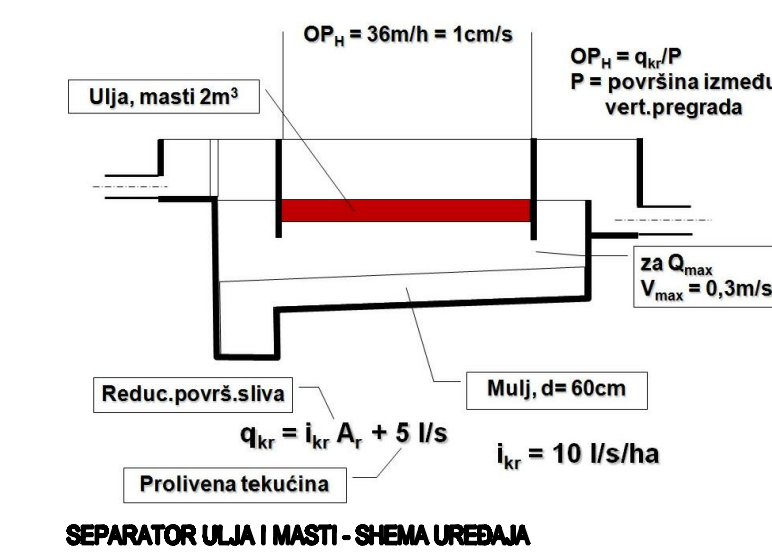
SEPARATOR ULJA I MASTI - ŠHEMA UREĐAJA
